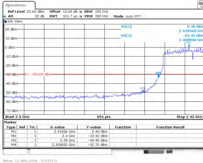
11AX40SISO_Ant1_Low_2422
