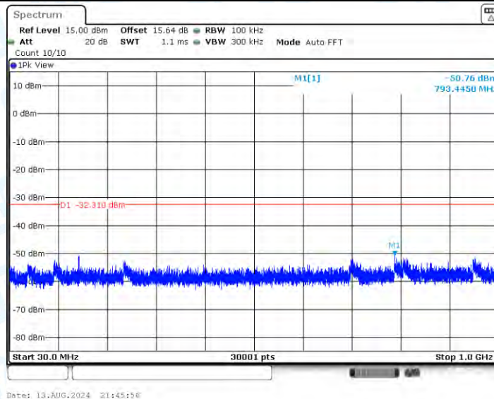
11AX40SISO_Ant1_2452_30~1000
