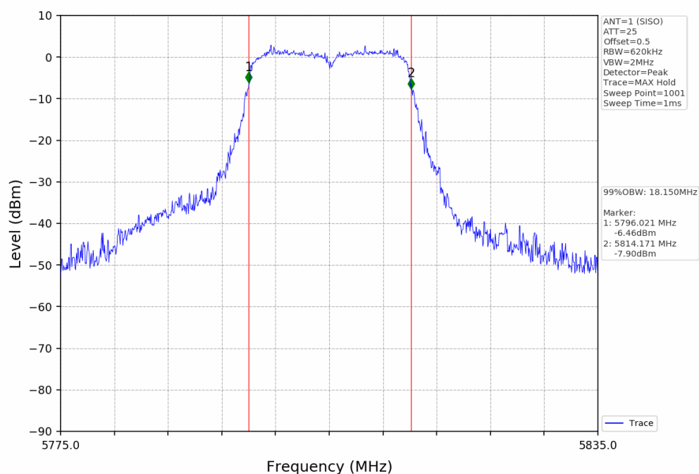
Bandwidth NTN 802.11n(HT20) SISO 5805MHz ANT1
