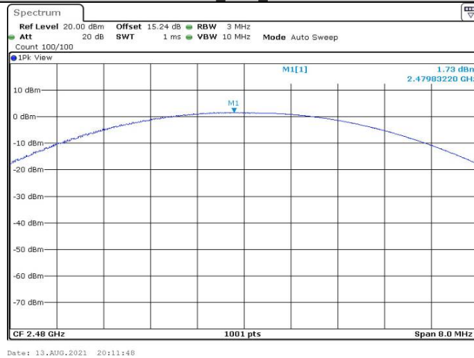
DH1_Ant1_2480
