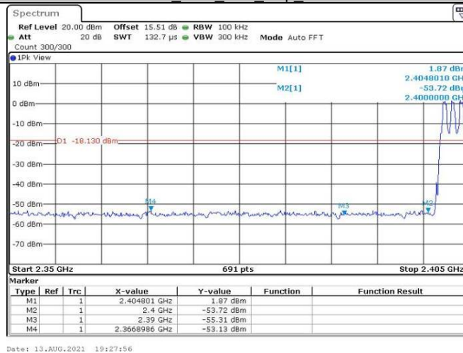
DH1_Ant1_Low_Hop_2402
