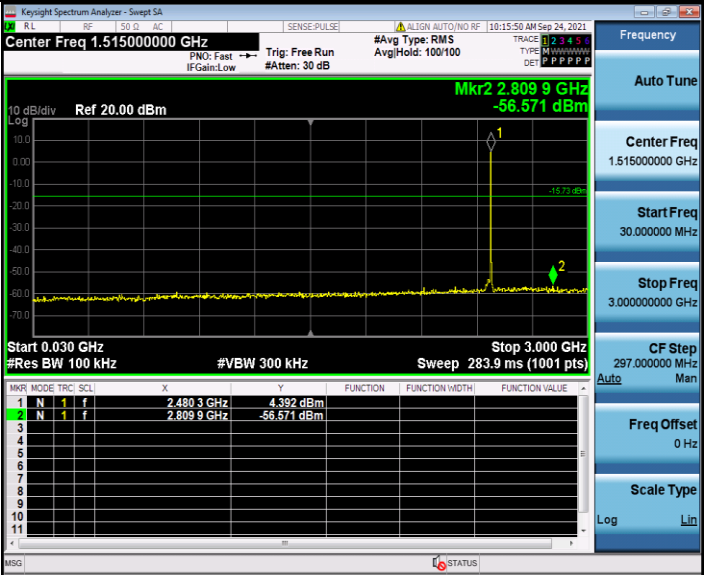
BLE_2480_30-3000
