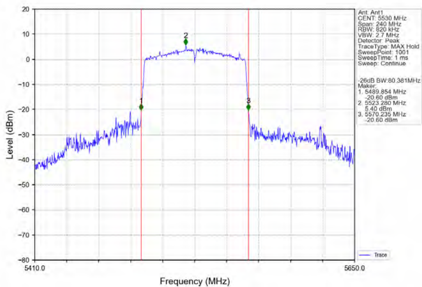
802.11ac(VHT80)_LCH_5530MHz_Ant1_NTNV
