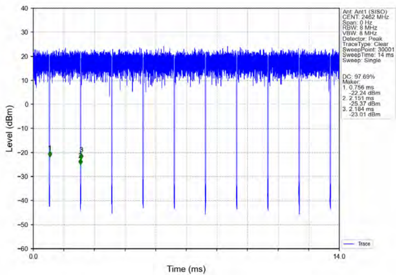
802.11g_HCH_2462MHz_Ant1 (SISO)_NTNV
