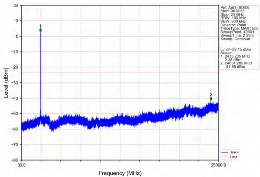
802.11g_MCH_2437MHz_Ant1 (SISO)_NTNV
