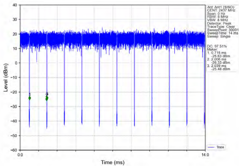
802.11n(HT20)_MCH_2437MHz_Ant1 (SISO)_NTNV
