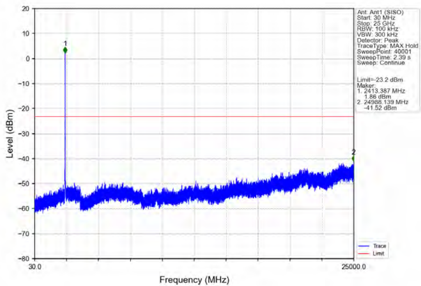
802.11n(HT20)_LCH_2412MHz_Ant1 (SISO)_NTNV
