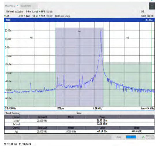
Band48-20MHz-QPSK-55990-1RB#99-PASS
