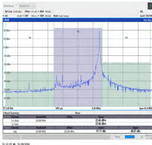
Band48-20MHz-QPSK-56640-1RB#99-PASS
