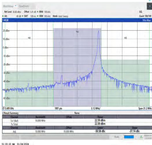
Band48-10MHz-QPSK-56690-1RB#49-PASS
