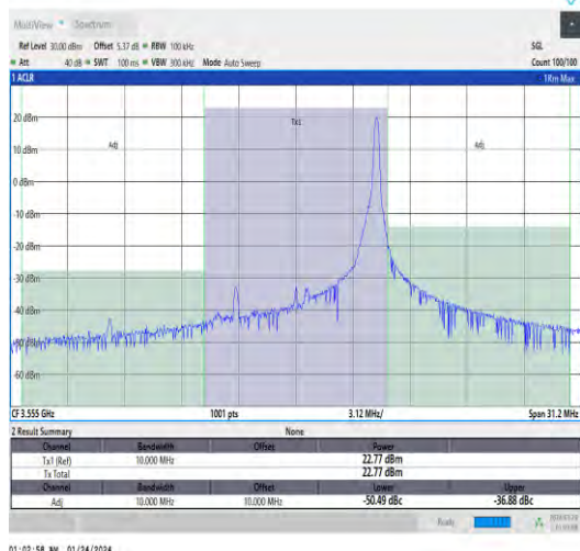
Band48-10MHz-QPSK-55290-1RB#49-PASS
