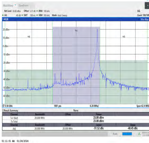
Band48-20MHz-QPSK-55340-1RB#99-PASS
