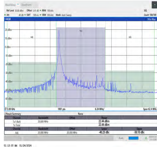
Band48-20MHz-QPSK-56640-1RB#0-PASS
