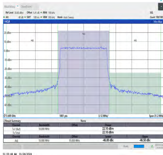
Band48-10MHz-QPSK-56690-50RB#0-PASS
