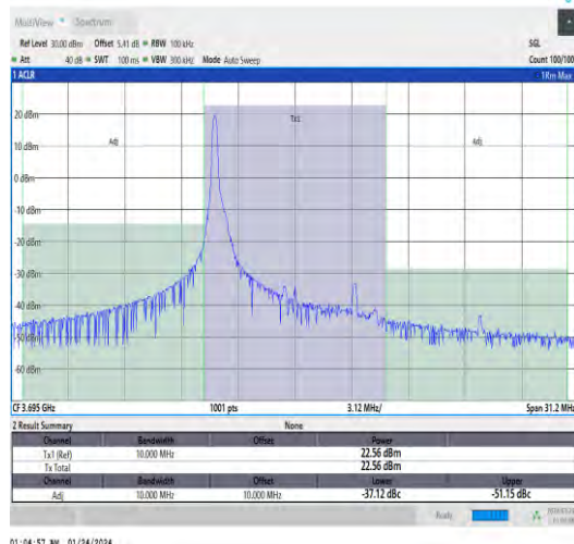
Band48-10MHz-QPSK-56690-1RB#0-PASS
