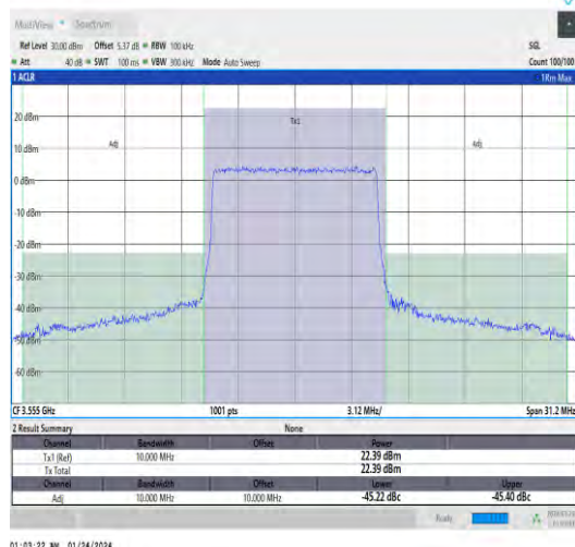
Band48-10MHz-QPSK-55290-50RB#0-PASS
