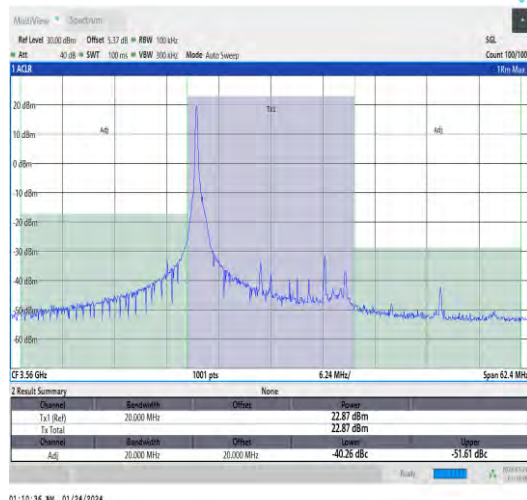
Band48-20MHz-QPSK-55340-1RB#0-PASS
