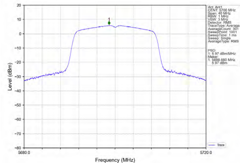
802.11ac(VHT20)_HCH_5700MHz_Ant1_NTNV
