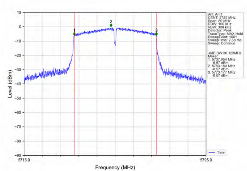
802.11ac(VHT40)_LCH_5755MHz_Ant1_NTNV
