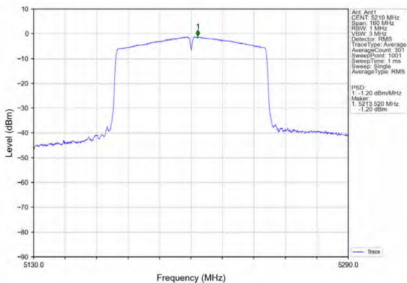
802.11ac(VHT80)_MCH_5210MHz_Ant1_NTNV
