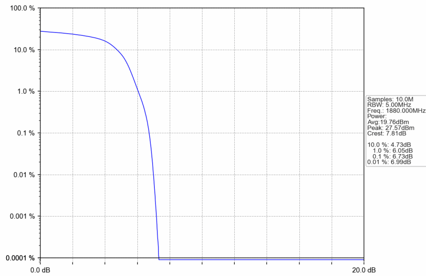
Band2_HSUPA_MCH_1880MHz_Subtest 1_NTNV
