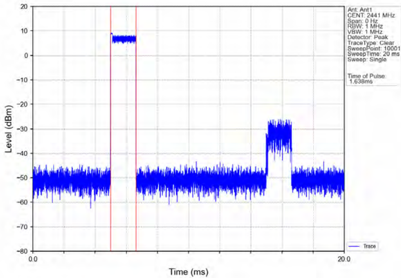
8DPSK_3DH3_HOPP_Ant1_NTNV
