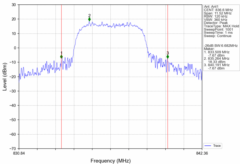
Band5_HSUPA_MCH_836.6MHz_Subtest 1_NTNV
