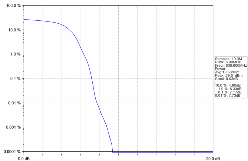
Band5_HSUPA_MCH_836.6MHz_Subtest 1_NTNV
