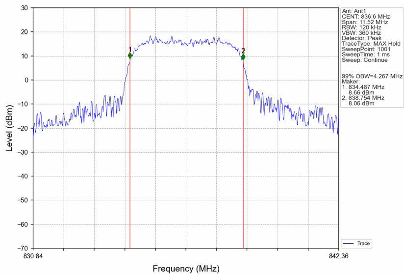
Band5_HSUPA_MCH_836.6MHz_Subtest 1_NTNV
