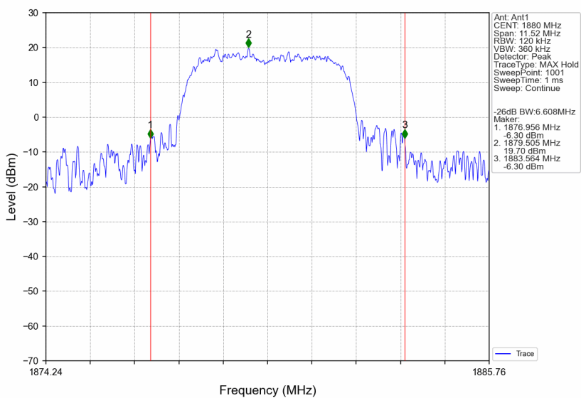
Band2_HSUPA_MCH_1880MHz_Subtest 1_NTNV
