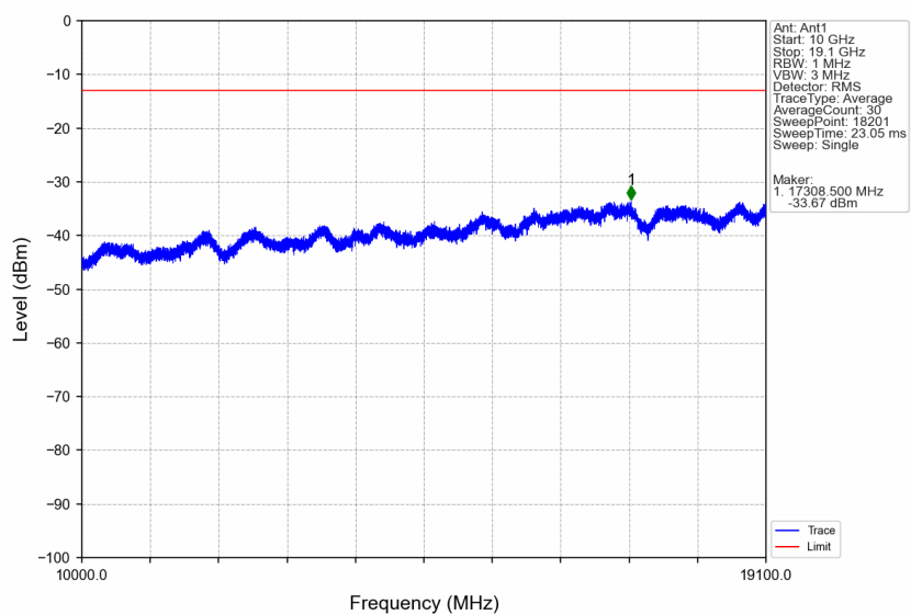
Band2_HSUPA_MCH_1880MHz_Subtest 1_NTNV
