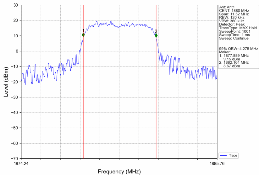
Band2_HSUPA_MCH_1880MHz_Subtest 1_NTNV
