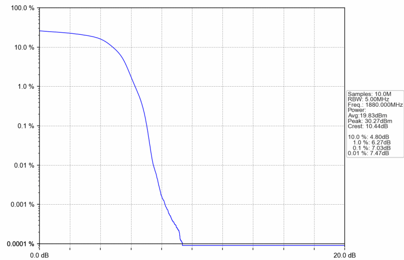
Band2_HSUPA_MCH_1880MHz_Subtest 1_NTNV
