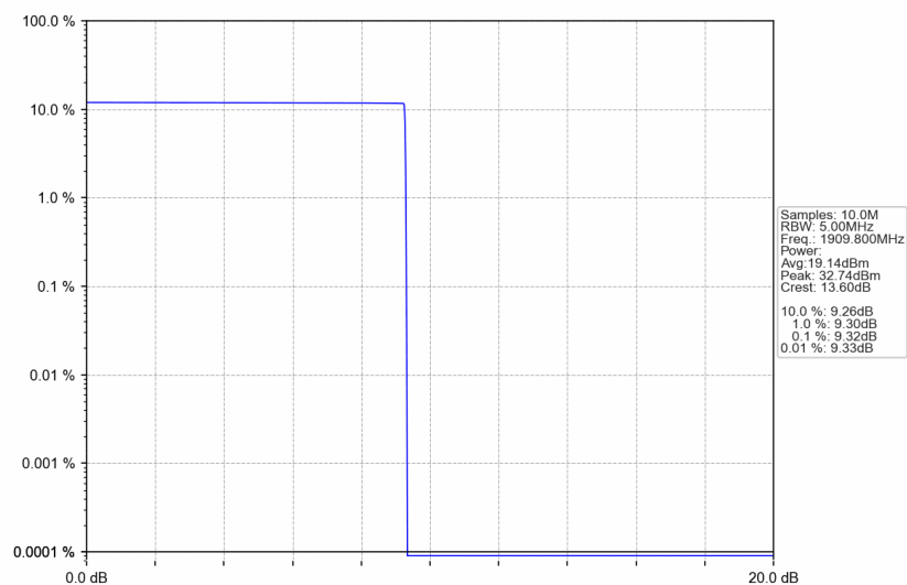
PCS1900 GSM_HCH_1909.8MHz_GSM_NTNV
