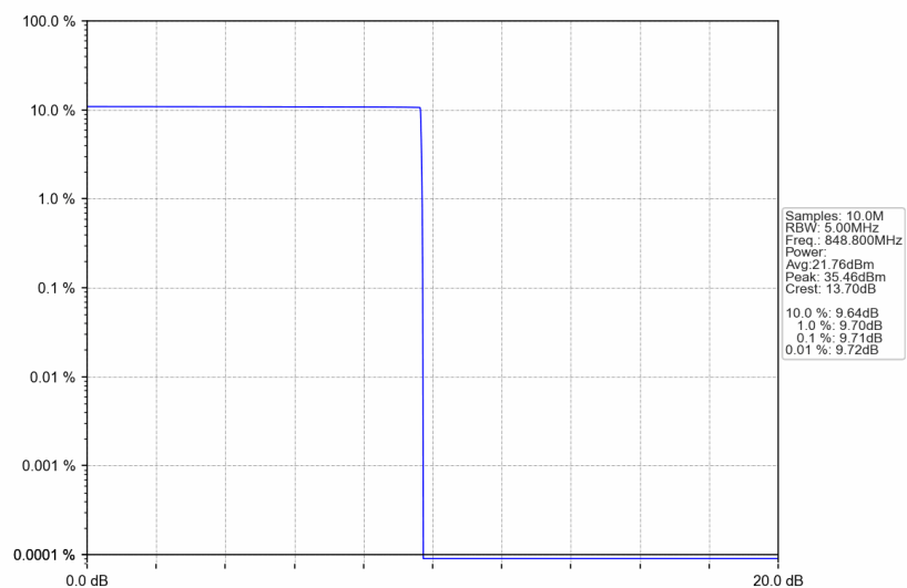
GSM850_GSM_HCH_848.8MHz_GSM_NTNV
