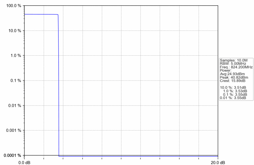
GSM850_GPRS_LCH_824.2MHz_4 TX Slots_NTNV
