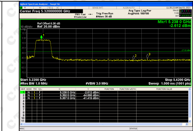
802.11n(HT40)-5230
