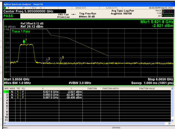
802.11(n20)-5825
