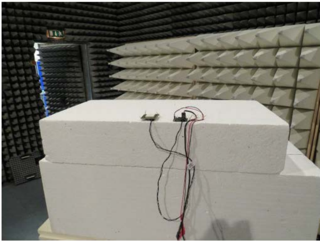
Setup EUT horizontal
