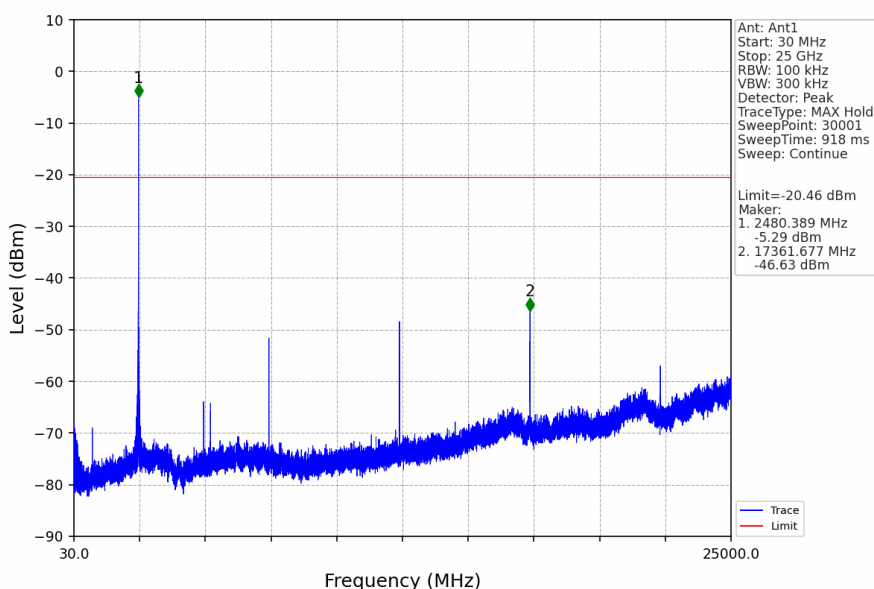
2M_HCH_2480MHz_Ant1_NTNV
