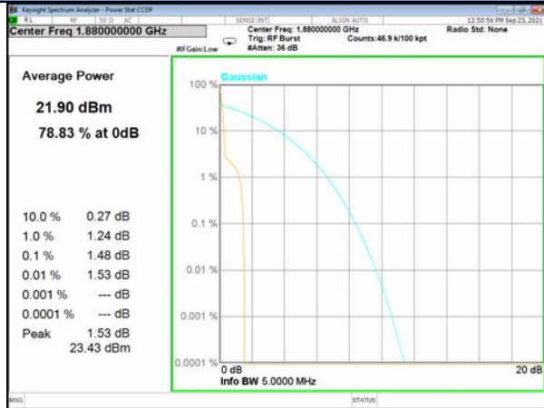
Band 2-15KHz-1#0-BPSK-Mid
