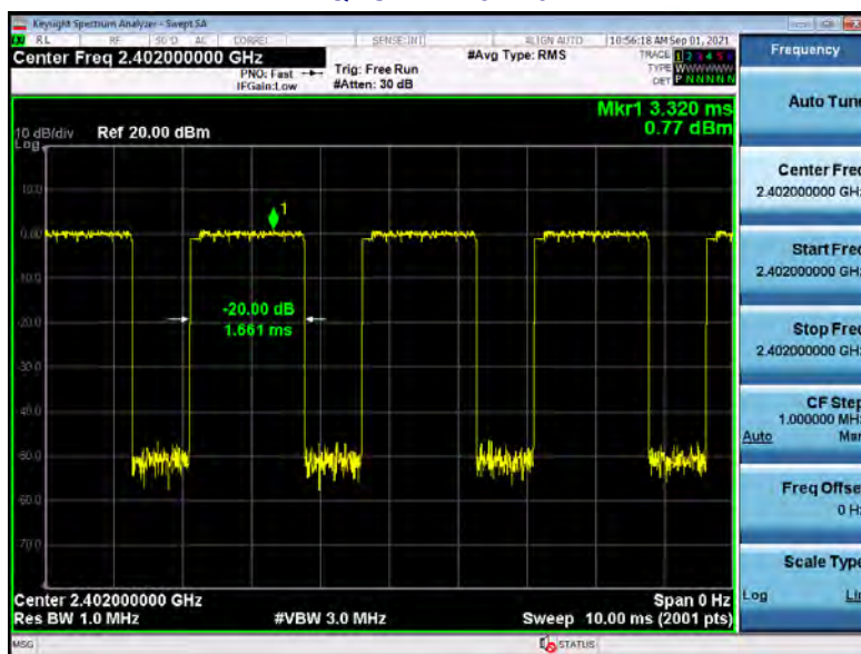
\pi/4 -DQPSK 2DH3 2402MHZ
