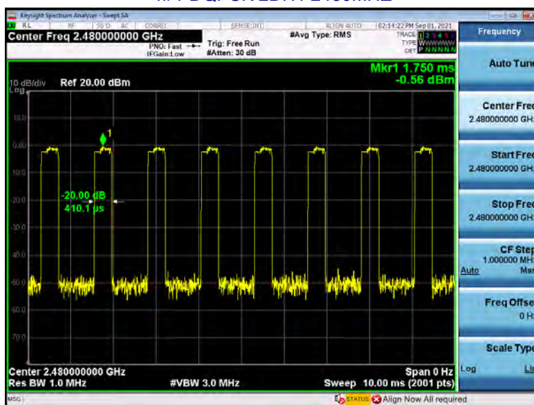
\pi/4 -DQPSK 2DH1 2480MHZ
