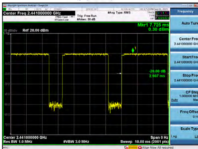
\pi/4 -DQPSK 2DH5 2441MHZ
