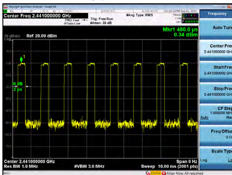
\pi/4 -DQPSK 2DH1 2441MHZ
