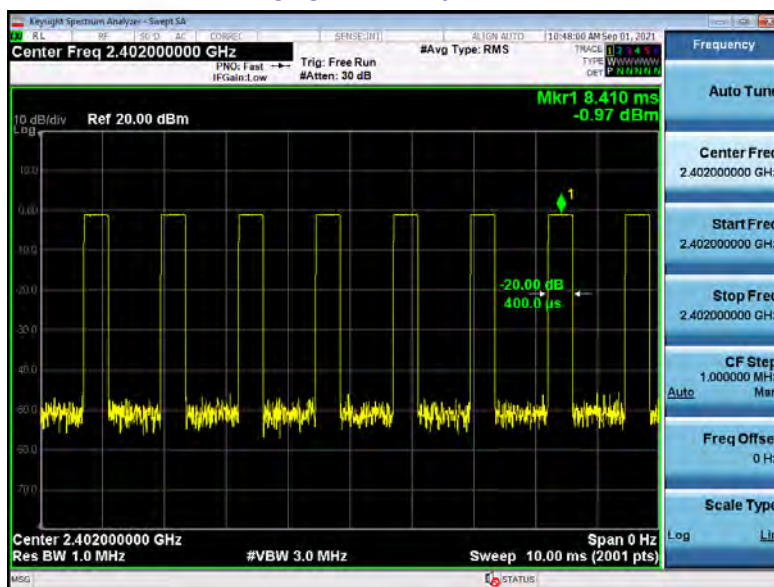
GFSK DH1 2402MHZ
