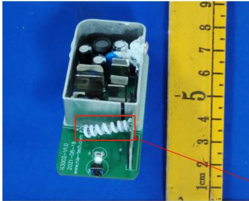
Antenna
