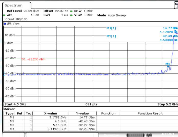
11AX40MIMO_Ant2_Low_5190_Peak
