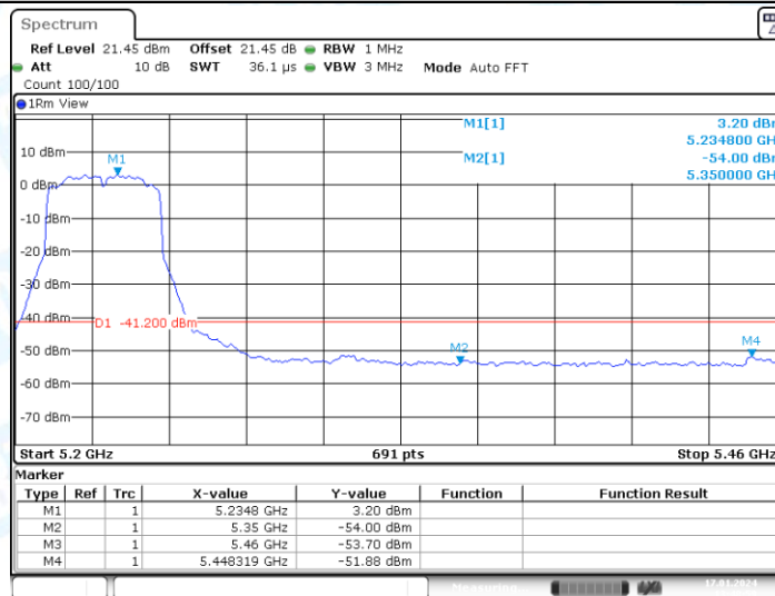
11AX40MIMO_Ant1_High_5230_AV
