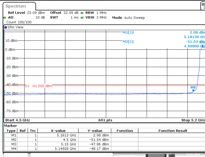
11AX40MIMO_Ant2_Low_5190_Peak
