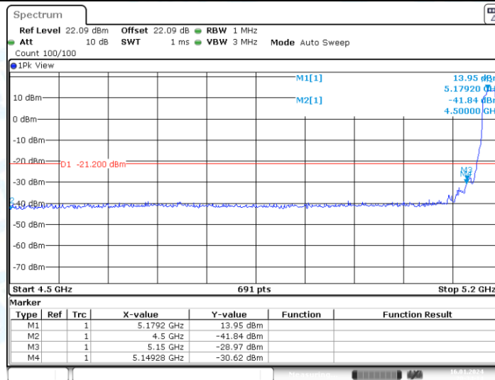
11N40MIMO_Ant2_Low_5190_Peak
