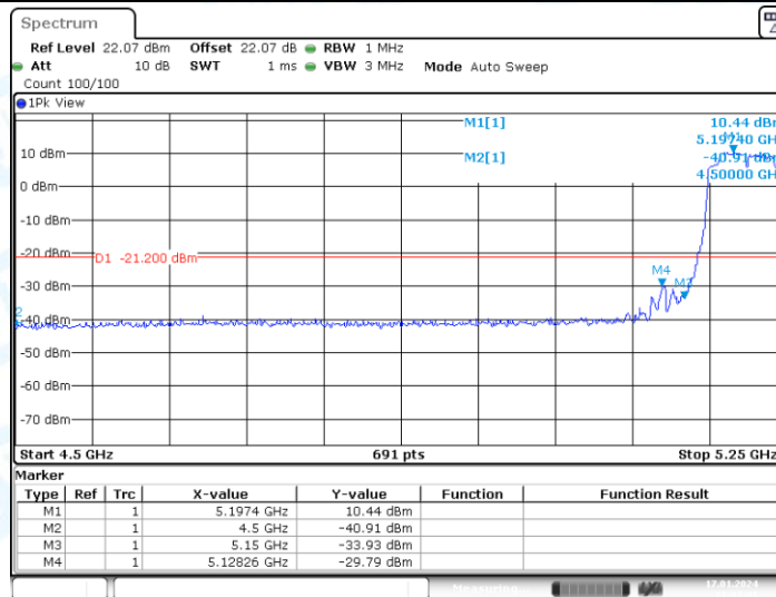
11AC80MIMO_Ant2_Low_5210_Peak
