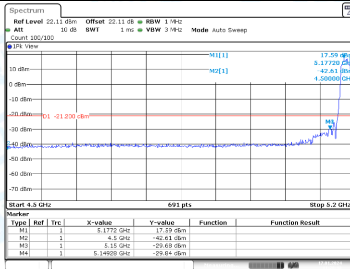
11AX20MIMO_Ant2_Low_5180_Peak
