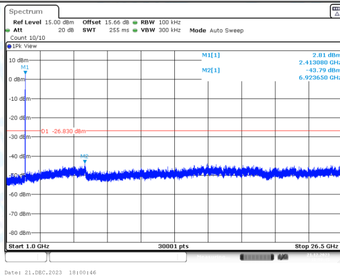
11AX20MIMO_Ant2_2412_0~Reference
