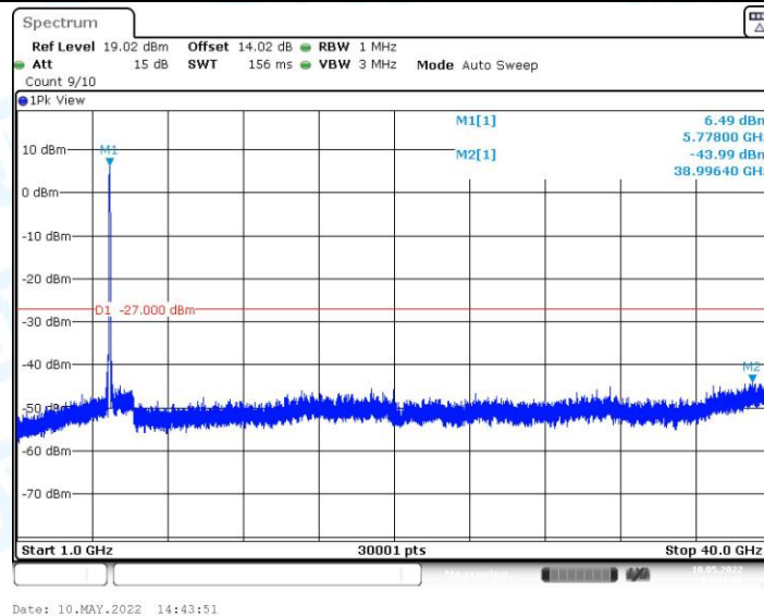
11AX80MIMO_Ant0_5775_1000~40000
