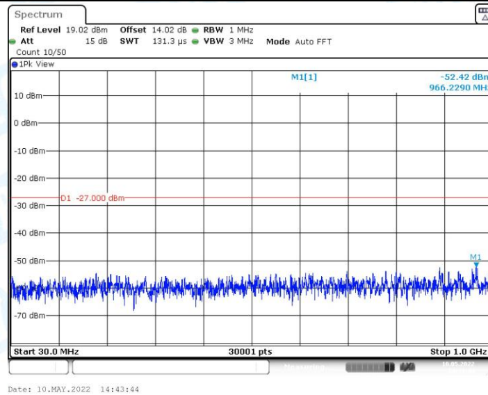
11AX80MIMO_Ant0_5775_30~1000
