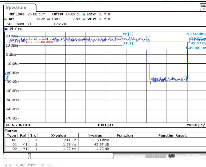
11AMIMO_Ant1_5785
