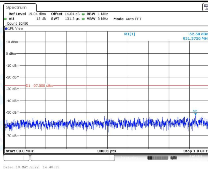
11AX80MIMO_Ant1_5775_30~1000
