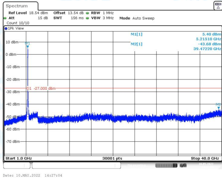
11AX80MIMO_Ant0_5210_1000~40000
