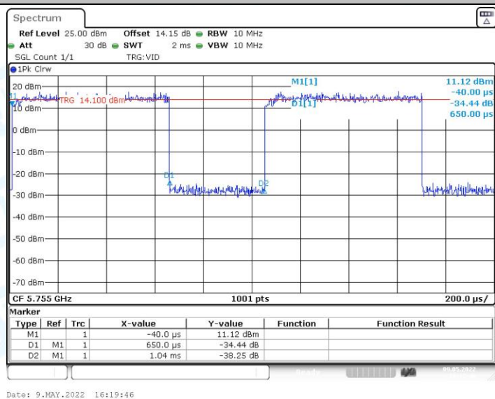
11N40MIMO_Ant0_5755
