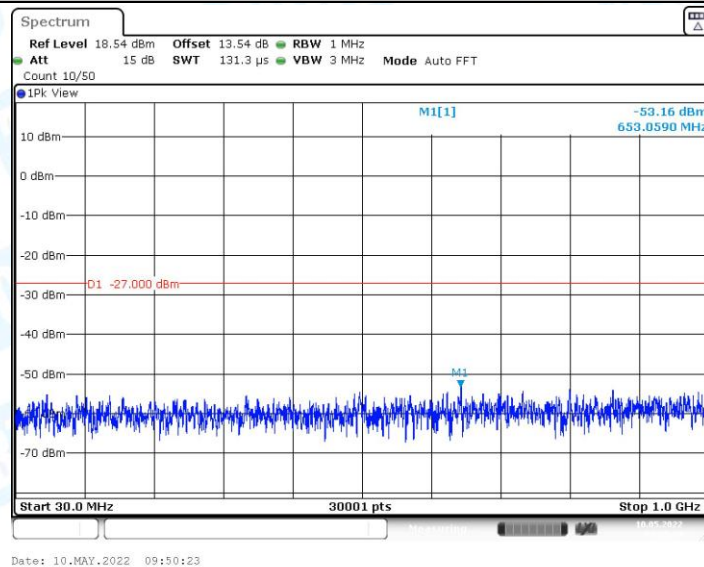
11AC80MIMO_Ant0_5210_30~1000
