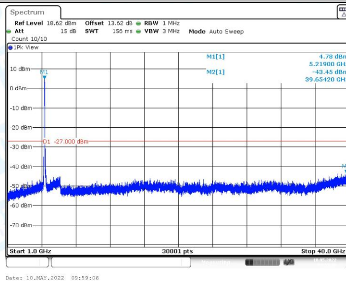
11AC80MIMO_Ant1_5210_1000~40000
