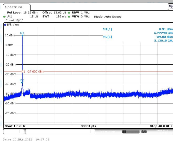
11AX20MIMO_Ant1_5220_1000~40000
