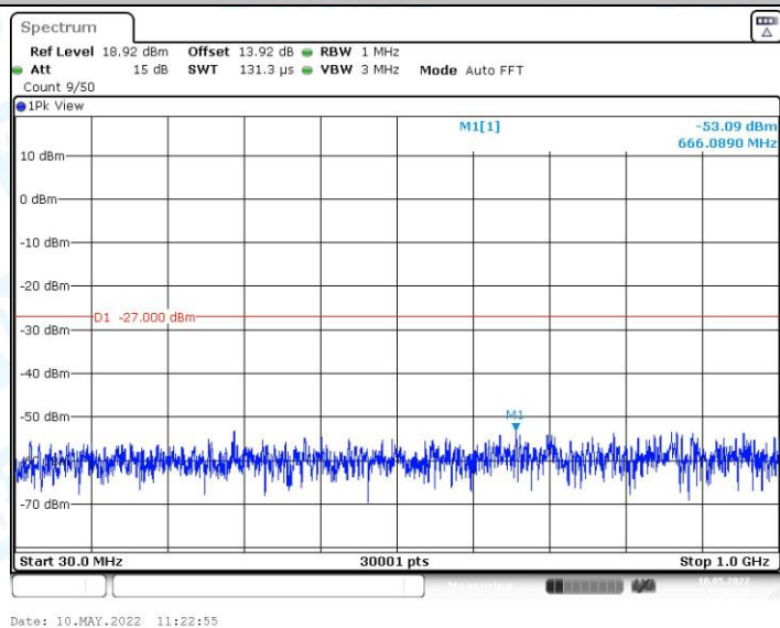
11AX20MIMO_Ant0_5785_30~1000
