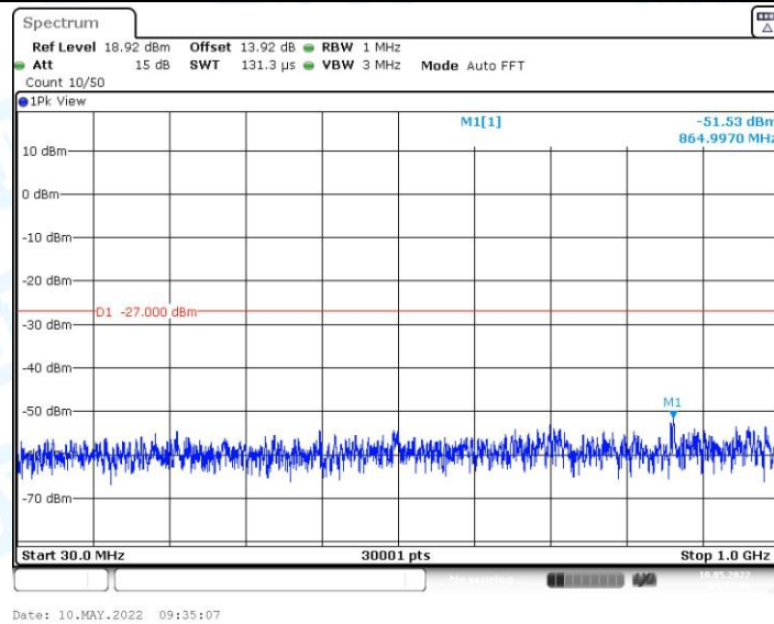
11AC40MIMO_Ant0_5795_30~1000
