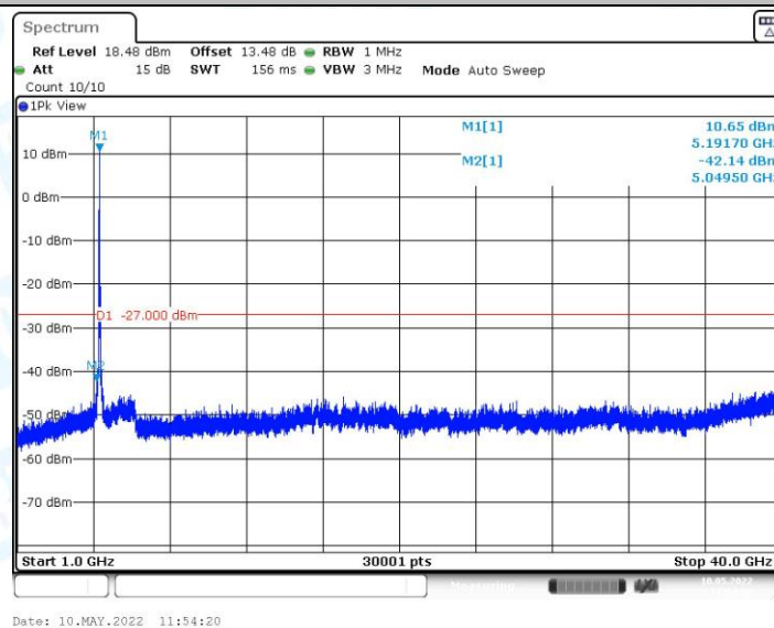
11AX40MIMO_Ant0_5190_1000~40000
