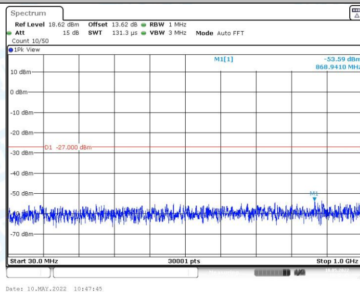
11AX20MIMO_Ant1_5220_30~1000
