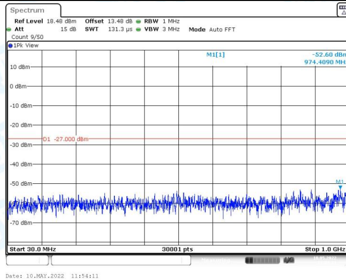
11AX40MIMO_Ant0_5190_30~1000
