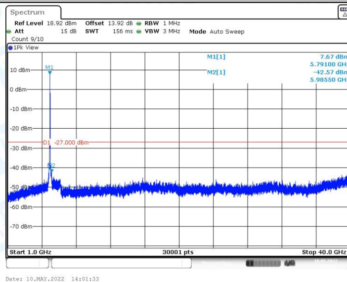
11AX40MIMO_Ant0_5795_1000~40000
