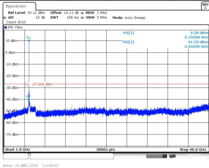
11AX20MIMO_Ant1_5745_1000~40000
