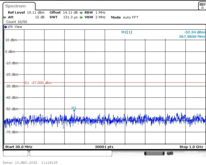
11AX20MIMO_Ant1_5745_30~1000
