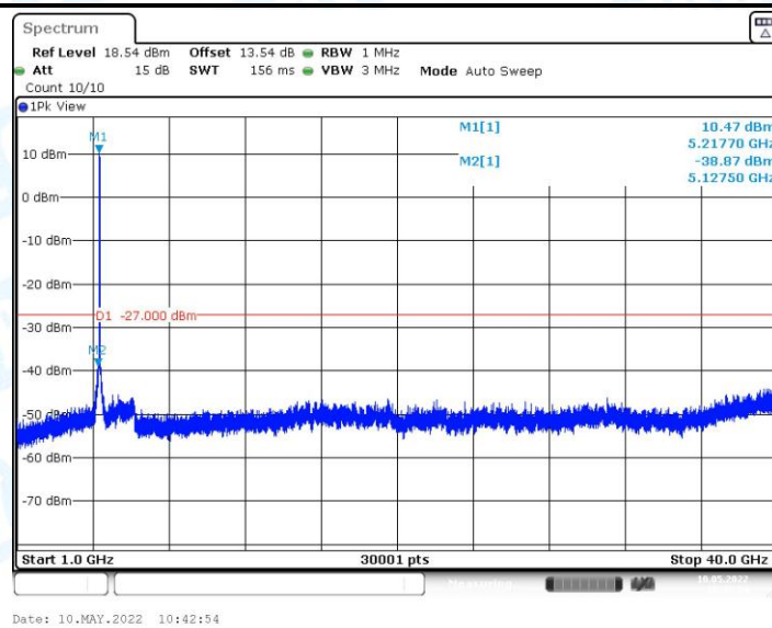
11AX20MIMO_Ant0_5220_1000~40000
