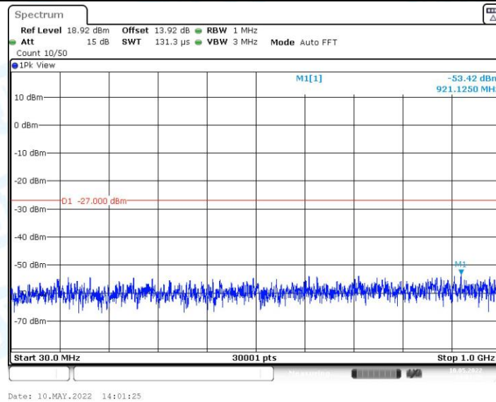
11AX40MIMO_Ant0_5795_30~1000
