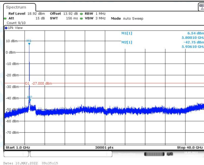
11AC40MIMO_Ant0_5795_1000~40000
