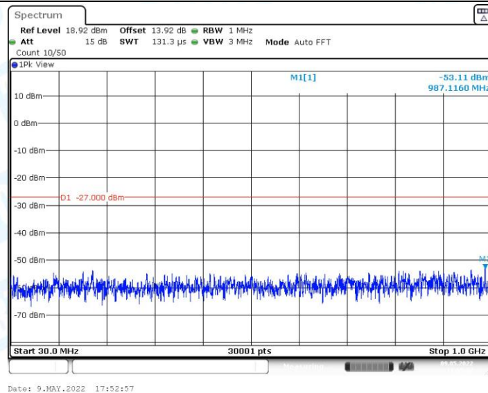
11AC20MIMO_Ant0_5785_30~1000
