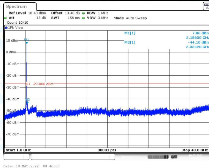
11AC40MIMO_Ant0_5190_1000~40000
