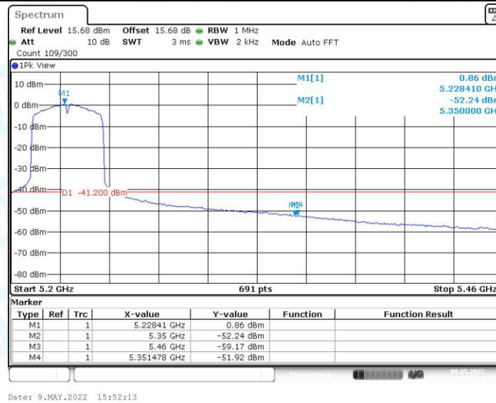
11N40MIMO_Ant0_High_5230_AV
