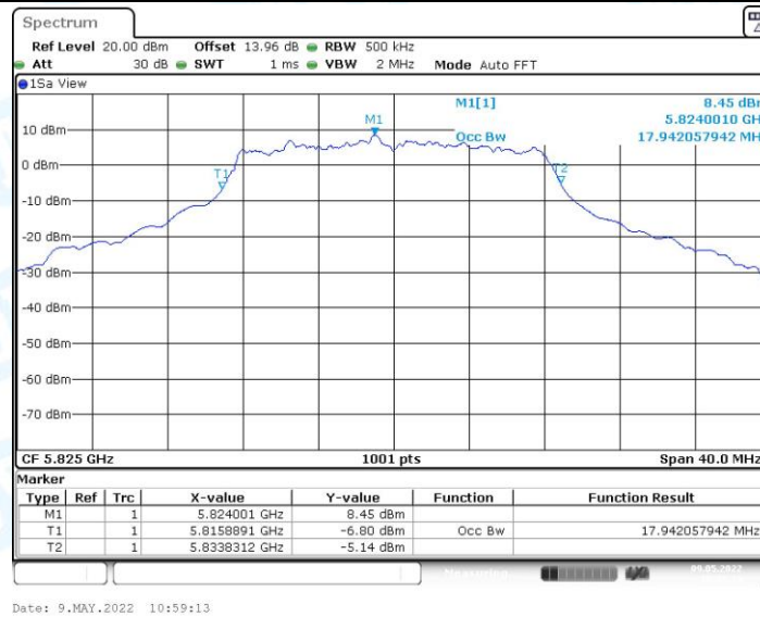
11AMIMO_Ant0_5825
