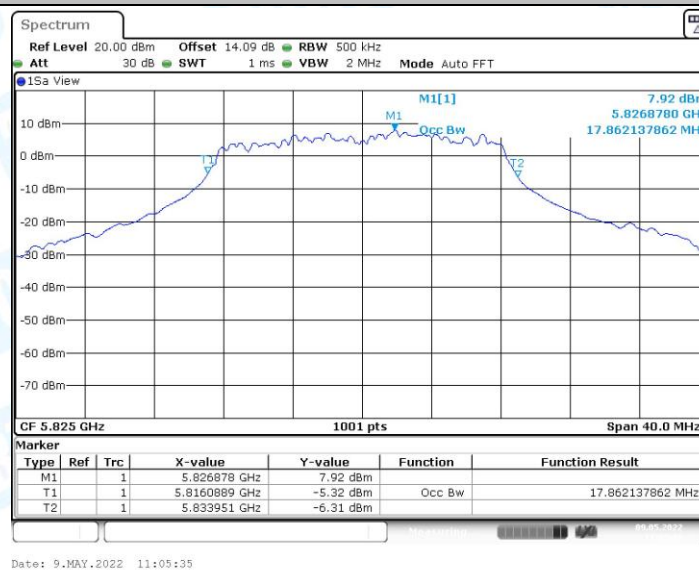
11AMIMO_Ant1_5825
