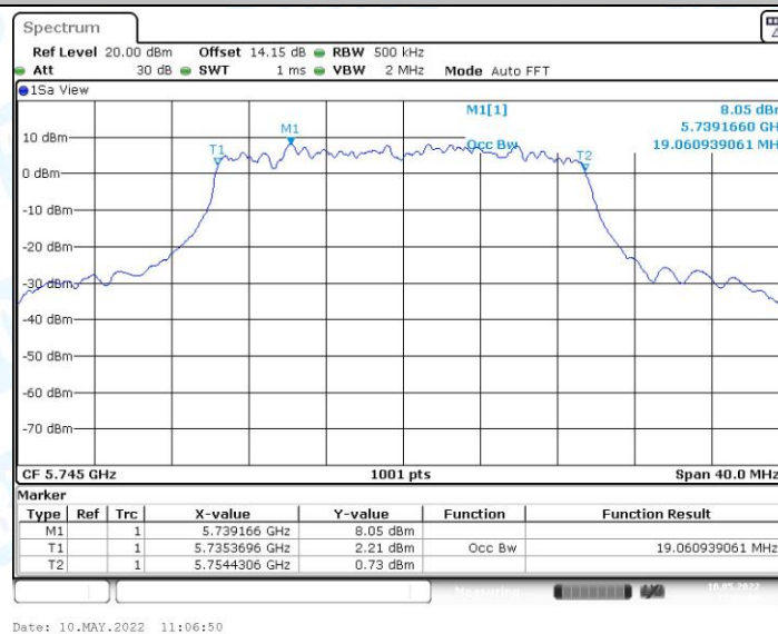
11AX20MIMO_Ant0_5745
