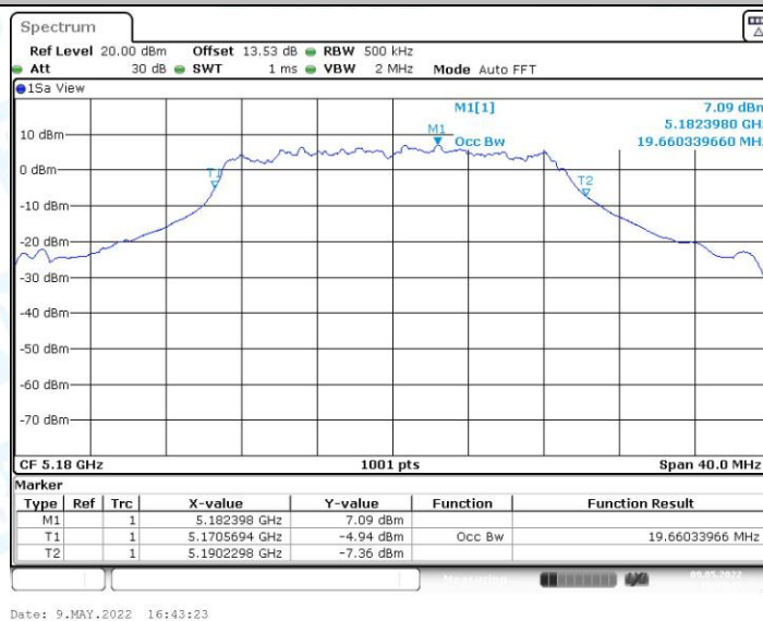
11AC20MIMO_Ant0_5180
