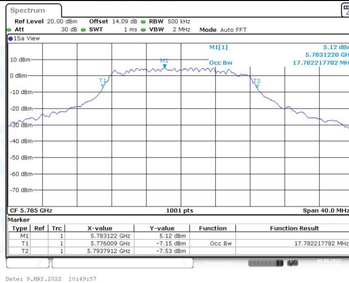
11AMIMO_Ant1_5785
