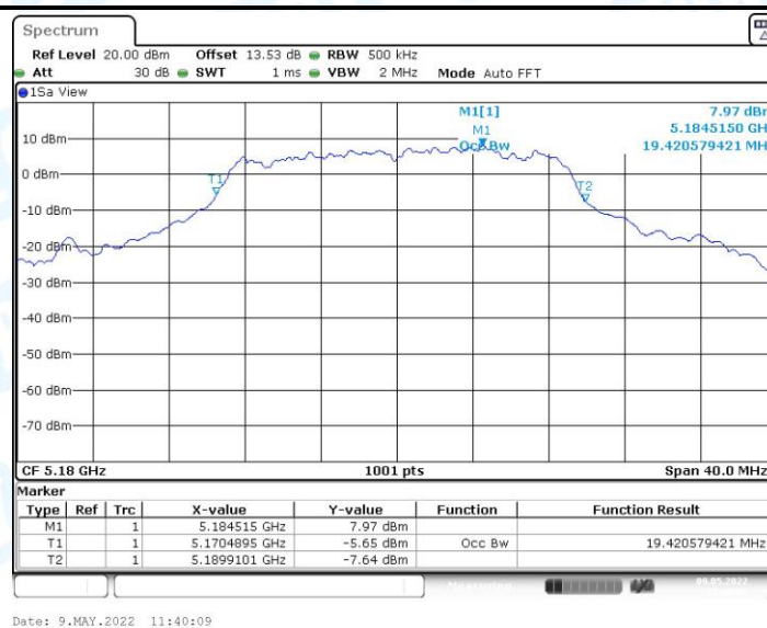
11N20MIMO_Ant0_5180
