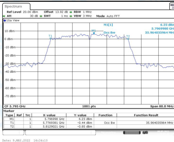
11N40MIMO_Ant0_5795
