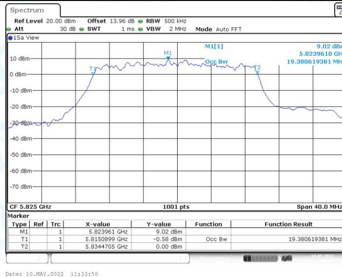
11AX20MIMO_Ant0_5825
