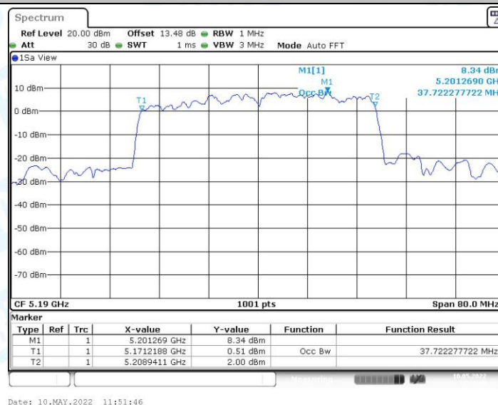
11AX40MIMO_Ant0_5190
