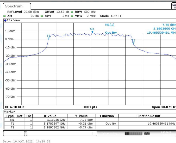
11AX20MIMO_Ant0_5180
