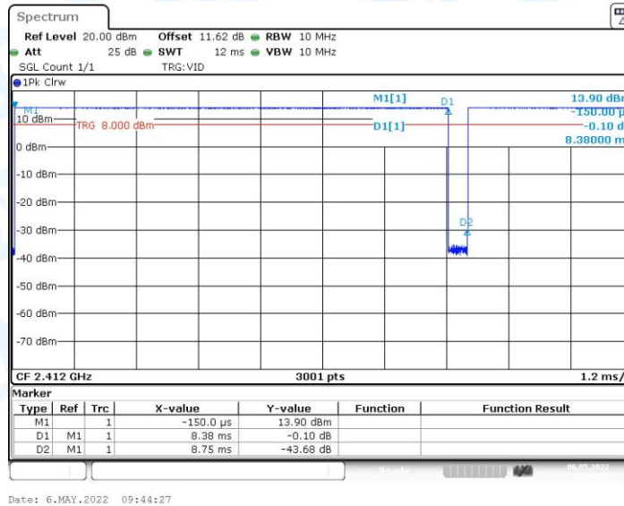
11BMIMO_Ant0_2412
