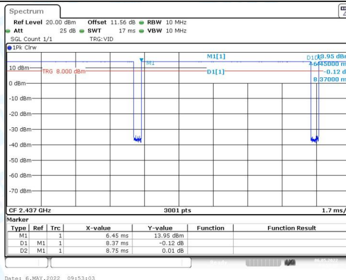
11BMIMO_Ant0_2437
