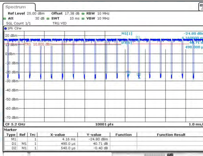
11AX20MIMO_Ant1_5200
