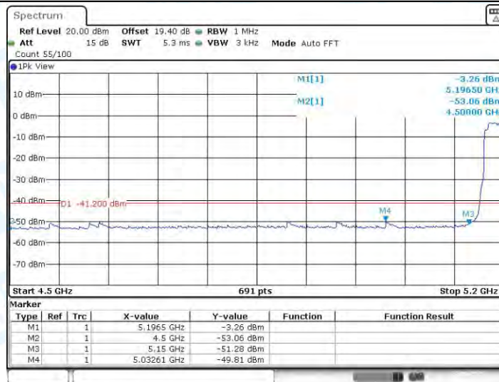
11N40MIMO_Ant1_Low_5190_AV
