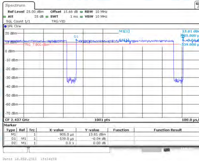
11AX20MIMO_Ant2_2437
