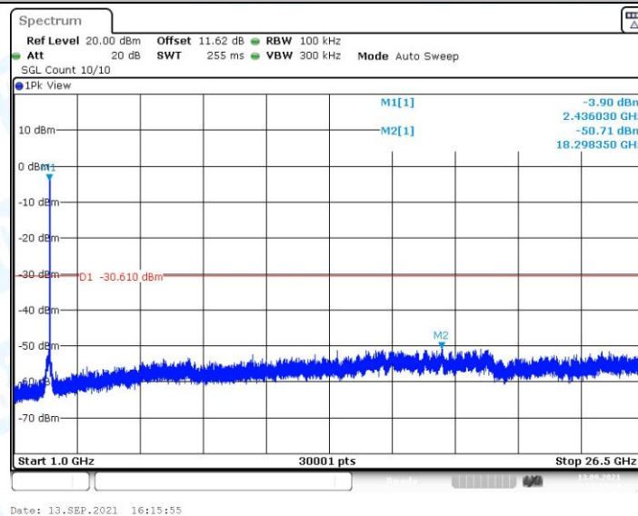
11G-CDD_Ant0_2437_1000~26500
