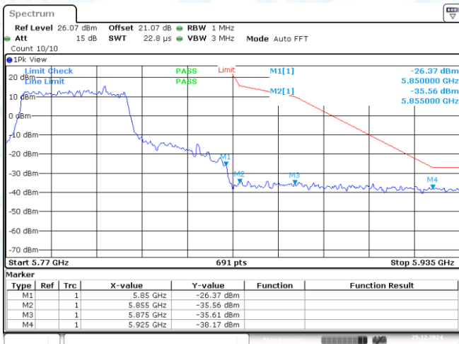
11AX40MIMO-Ant1-5755-PASS
