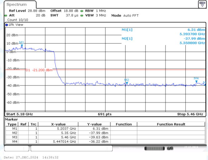
11AX80MIMO-Ant1-5210-PASS
