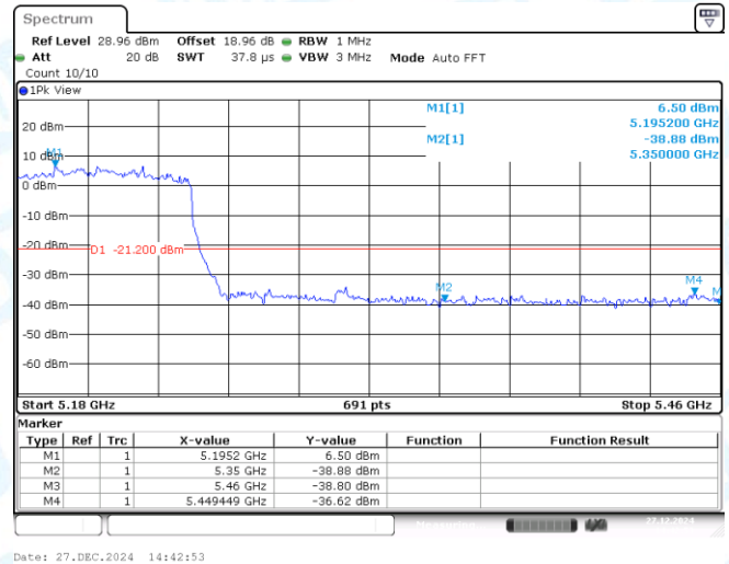
11AX80MIMO-Ant1-5210-PASS
