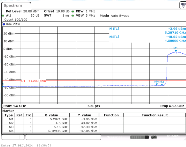
11AX80MIMO-Ant1-5210-PASS
