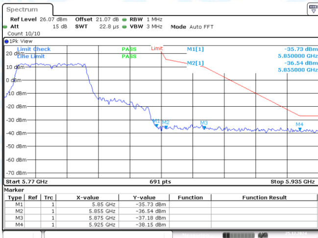
11N40MIMO-Ant1-5755-PASS
