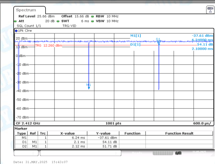
NTNV-11AX20MIMO-Ant1-2412
