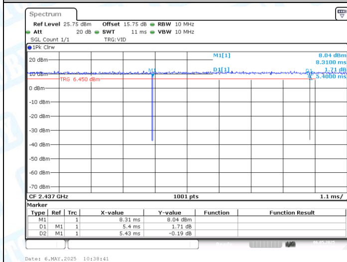
NTNV-11AX20MIMO-Ant2-2437
