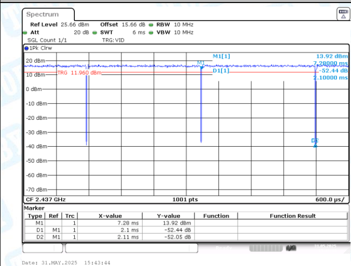
NTNV-11AX20MIMO-Ant1-2437
