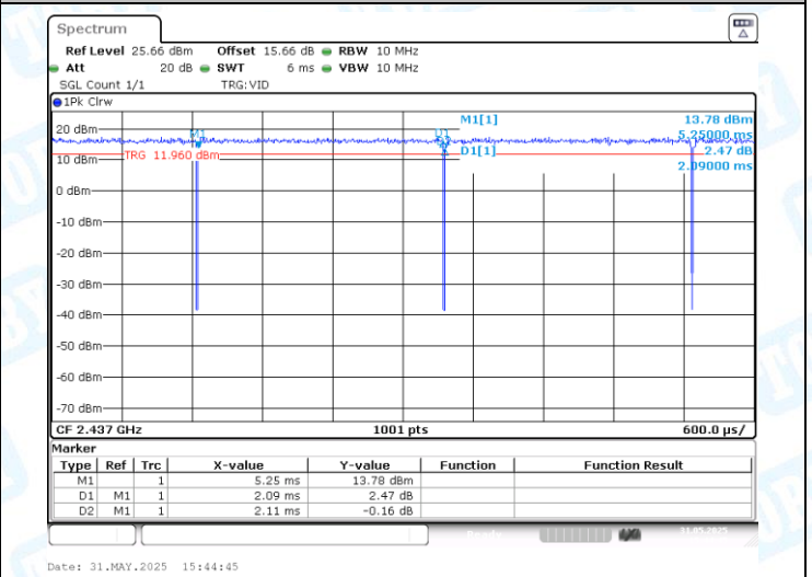
NTNV-11N40MIMO-Ant1-2437
