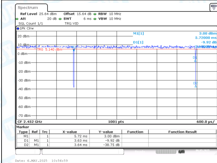
NTNV-11AX40MIMO-Ant1-2452
