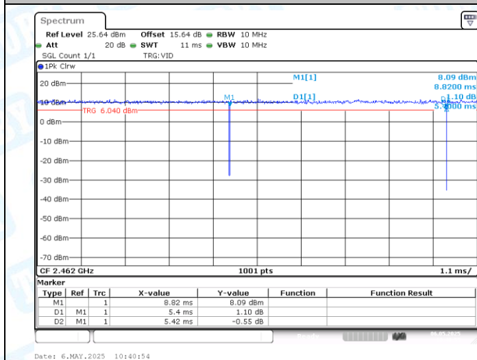
NTNV-11AX20MIMO-Ant1-2462
