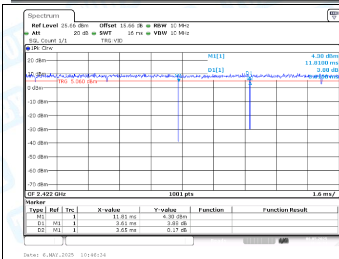
NTNV-11AX40MIMO-Ant1-2422
