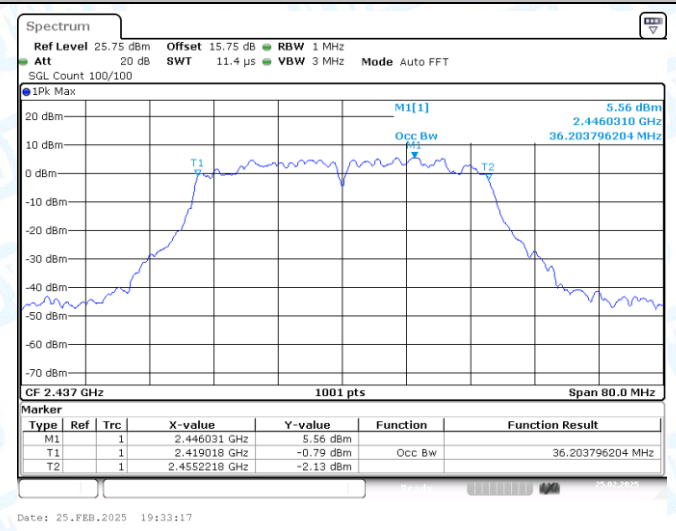
11N40MIMO-Ant2-2437
