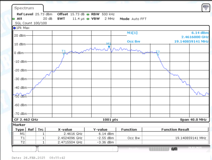
11AX20MIMO-Ant2-2462
