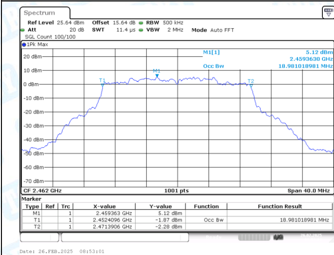
11AX20MIMO-Ant1-2462
