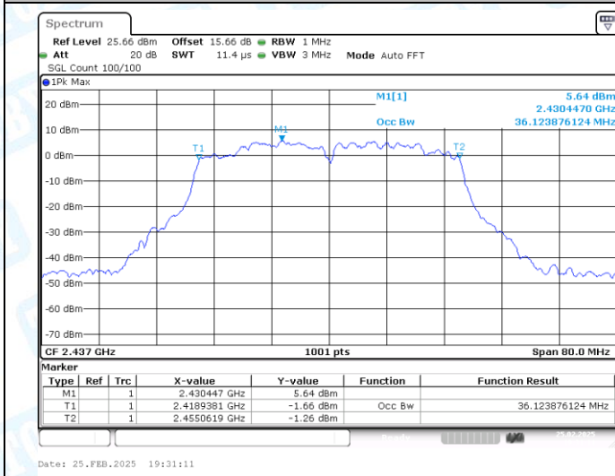
11N40MIMO-Ant1-2437
