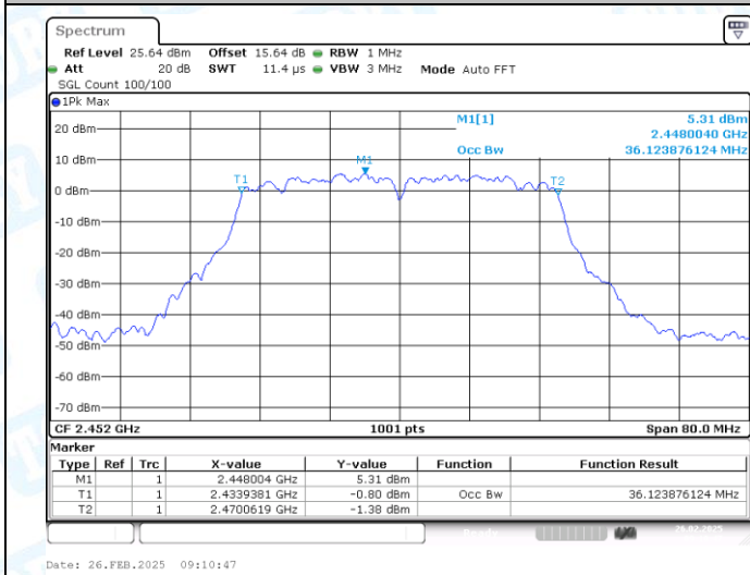
11AX40MIMO-Ant1-2452
