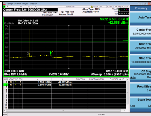
CATM1 B4-5M-High CH-CSE-2-QPSK-1 RB 0
