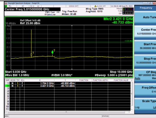
CATM1 B4-3M-Low CH-CSE-2-Q16-1 RB 0
