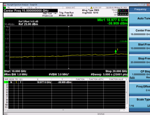
CATM1 B4-10M-Mid CH-CSE-1-Q16-1 RB 0
