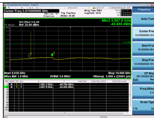
CATM1 B4-1.4M-High CH-CSE-2-Q16-1 RB 0
