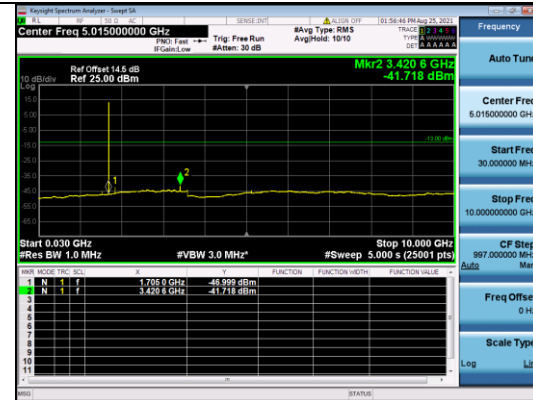
CATM1 B4-5M-Low CH-CSE-2-Q16-1 RB 0
