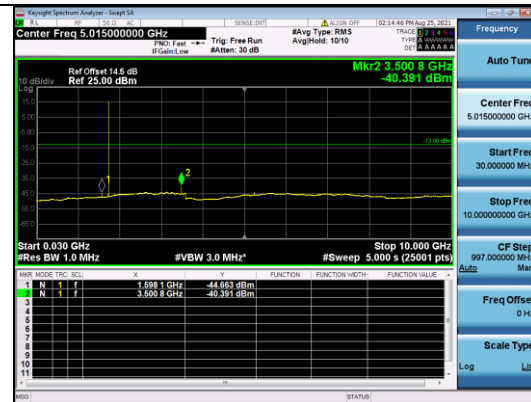
CATM1 B4-5M-High CH-CSE-2-Q16-1 RB 0
