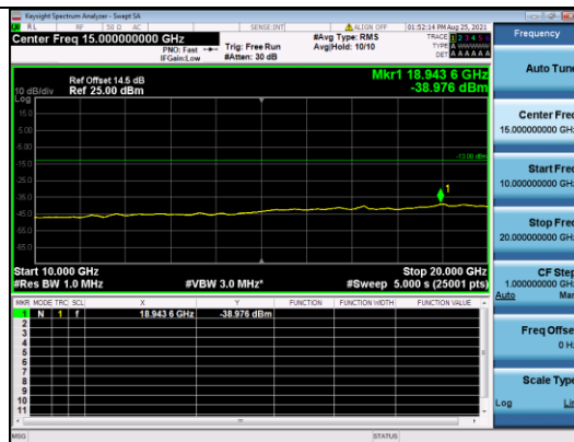
CATM1 B4-5M-Mid CH-CSE-1-QPSK-1 RB 0
