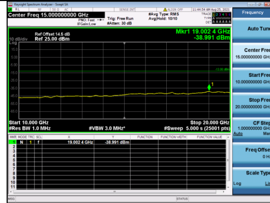
CATM1 B4-3M-High CH-CSE-1-Q16-1 RB 0
