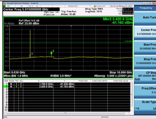
CATM1 B4-5M-Low CH-CSE-2-QPSK-1 RB 0
