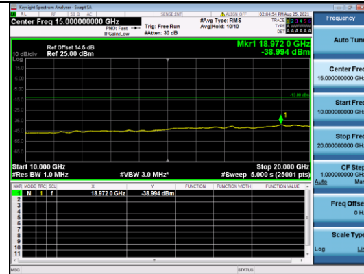
CATM1 B4-5M-High CH-CSE-1-Q16-1 RB 0
