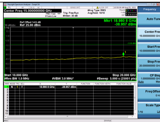
CATM1 B4-1.4M-High CH-CSE-1-Q16-1 RB 0
