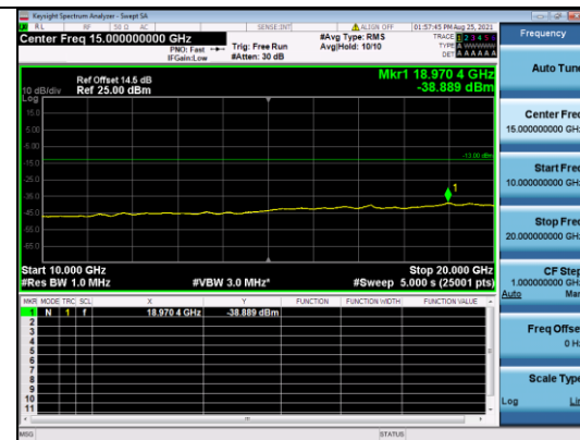
CATM1 B4-5M-Mid CH-CSE-1-Q16-1 RB 0
