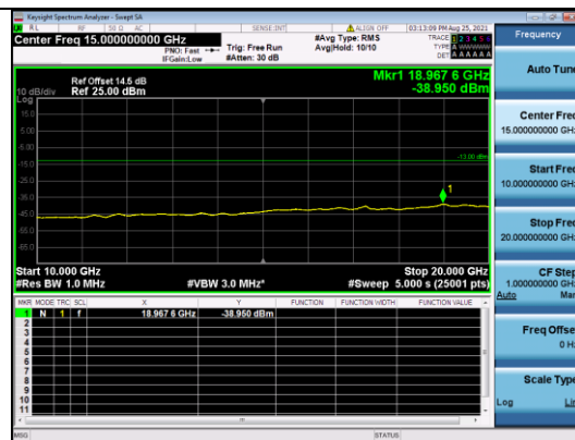
CATM1 B4-10M-High CH-CSE-2-Q16-1 RB 0
