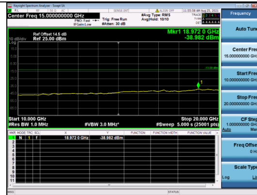
CATM1 B4-3M-High CH-CSE-2-Q16-1 RB 0
