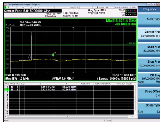
CATM1 B4-10M-Low CH-CSE-2-Q16-1 RB 0
