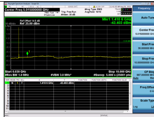
B12-5M-High CH-CSE-1-Q16-1 RB 0
