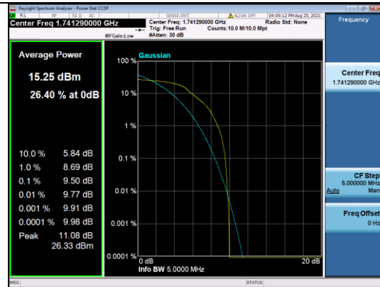
LTE CATM1 B4-15M-High CH-PAPR-Q16
