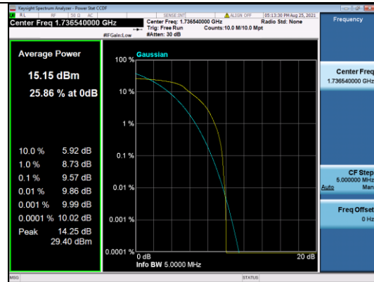
LTE CATM1 B4-20M-High CH-PAPR-Q16
