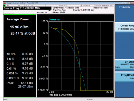
LTE CATM1 B12-3M-High CH-PAPR-Q16
