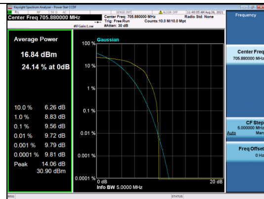
LTE CATM1 B12-5M-High CH-PAPR-Q16
