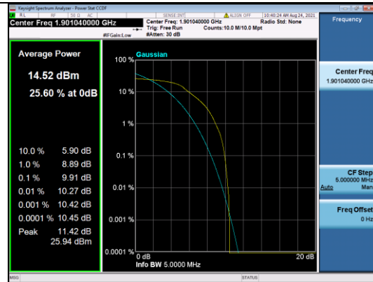
LTE CATM1 B2-10M-High CH-PAPR-Q16
