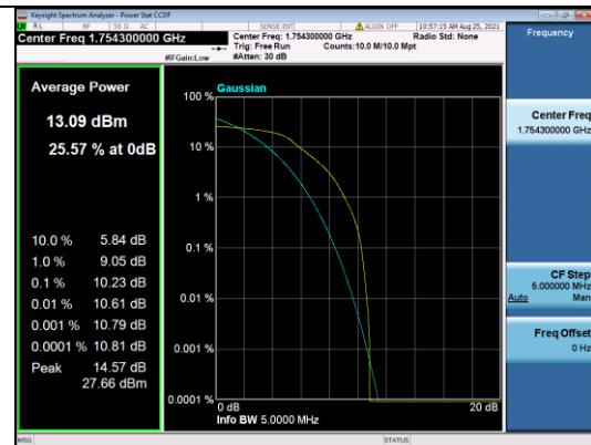
LTE CATM1 B4-1.4M-High CH-PAPR-Q16
