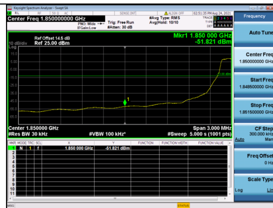
CATM1 B2-20M-Low CH-BE-Q16-1 RB 0
