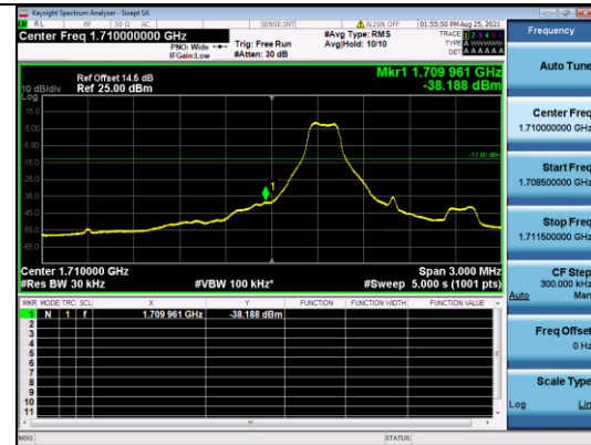
CATM1 B4-5M-Low CH-BE-Q16-1 RB 0
