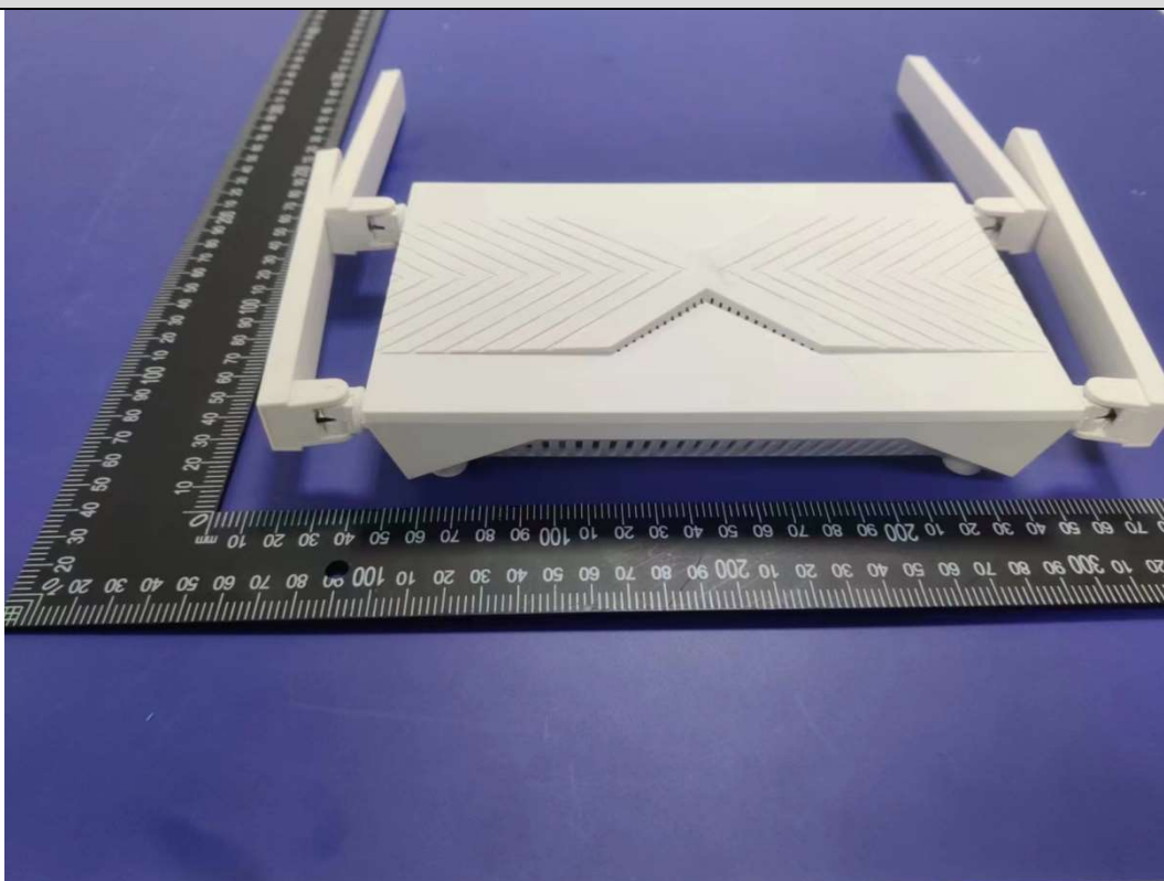
EUT5 Photo
