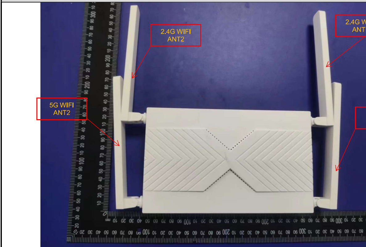
EUT5 Photo
