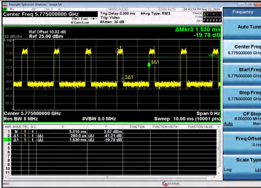
NTNV-11AX80SISO-Ant1-5775
